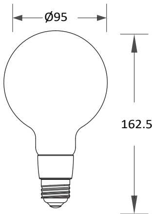
燈頭：E27
