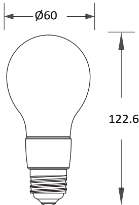
燈頭：E27
