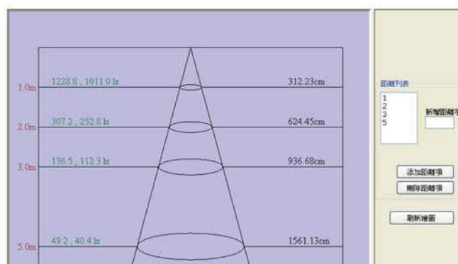
LED-T361-0845W 照度距離圖表
