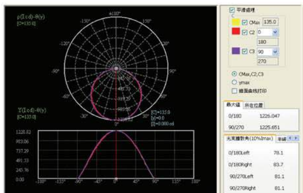
LED-T361-0845W 光強分佈曲線
