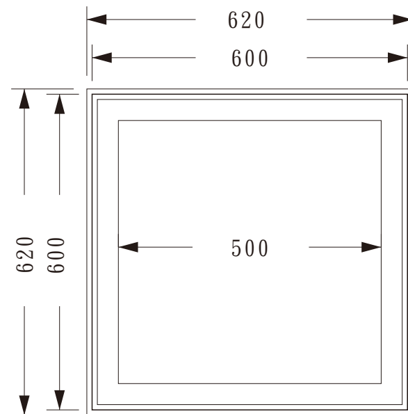
鑄鐵框正面圖
