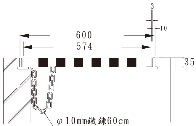
框蓋剖面圖
