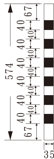
A-A剖面圖
