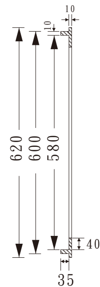
框剖面圖
