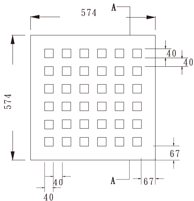
鑄鐵蓋平面圖
