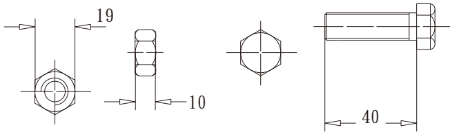
螺絲螺帽詳圖
