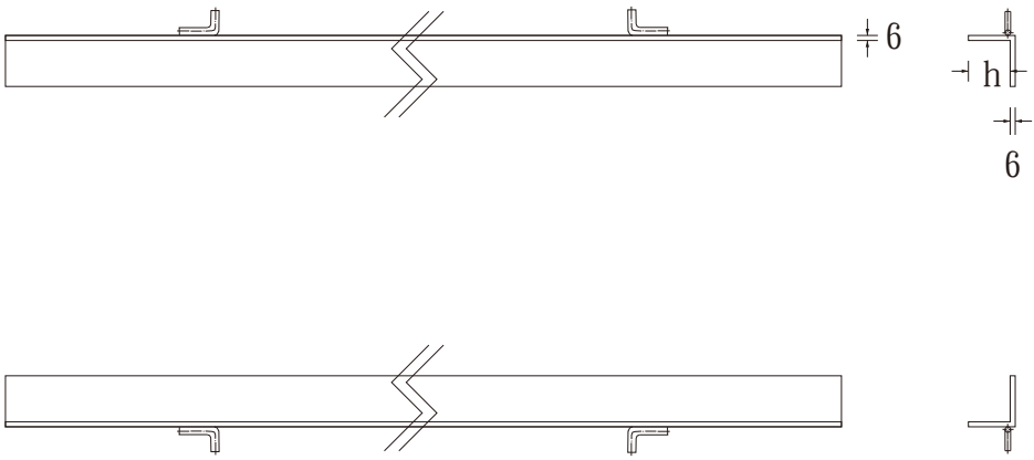
連續型框座詳圖
