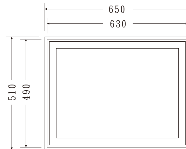
鑄鐵框
