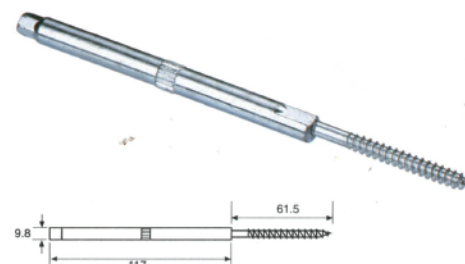
CH18 隱藏式層板螺絲
