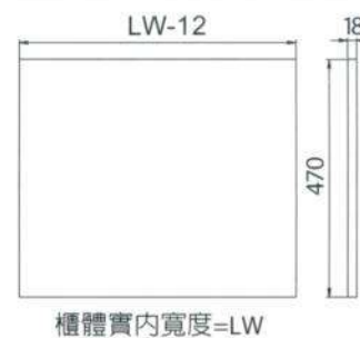
輔助檯面尺寸圖 Counter top Template
