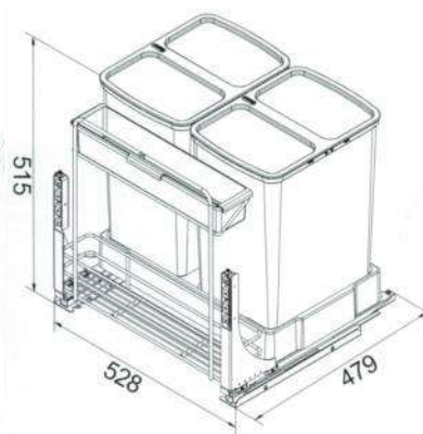
示意圖 / 門板孔位圖 Schematic / Door Hole Location Diagram
