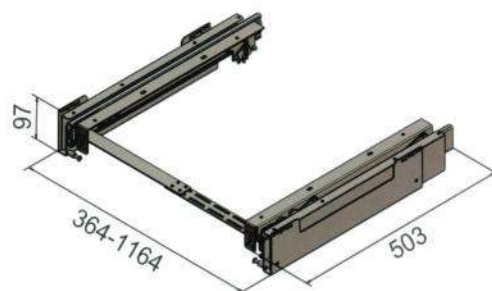
輔助檯面尺寸圖 Counter top Template
