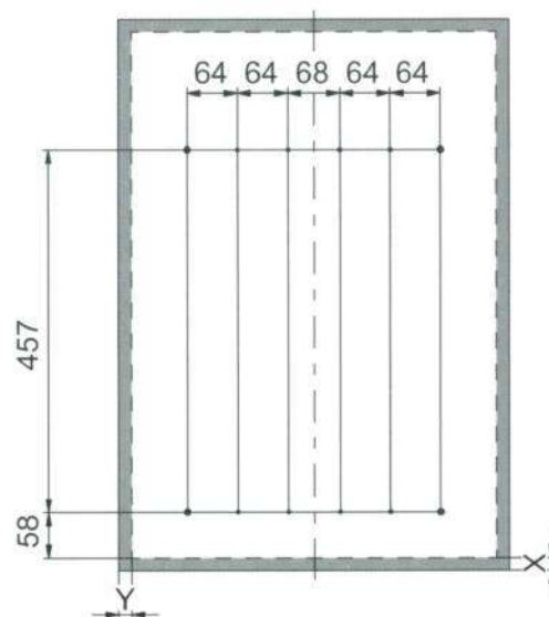
門板孔位圖 Door Panel Schematic
