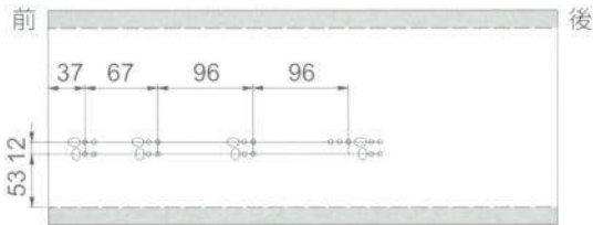
滑軌孔位示意圖
