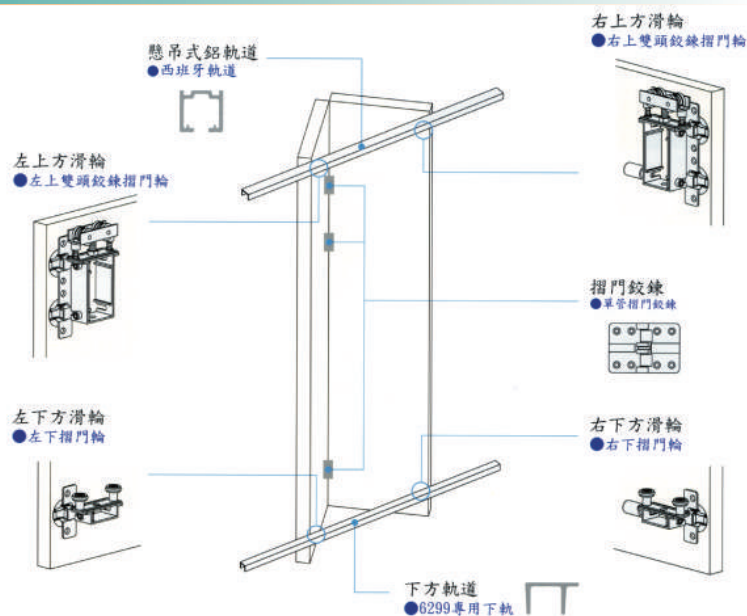
※組合成摺門所需五金配件
