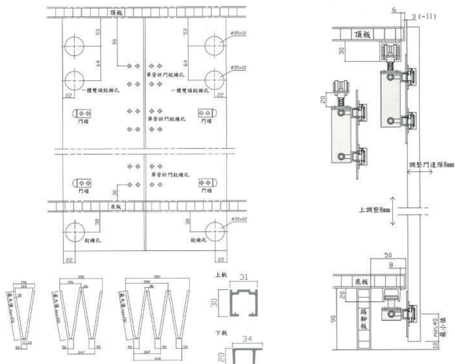
蓋柱摺門安裝示意圖
