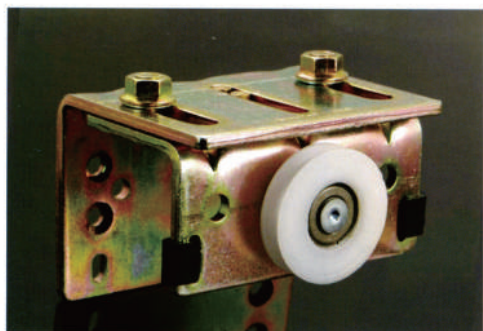
6298 外蓋推拉門-木門
