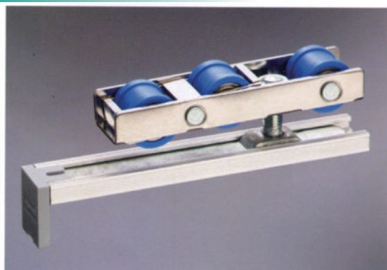
西班牙重型吊輪(平衡式)
