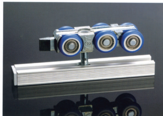
797無縫重型輪(平衡式)
