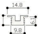
T型下軌 材質：鋁合金 顏色：鋁本色、古銅、金色
