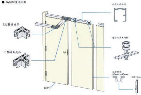
● 隔間配置示意圖
