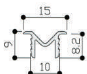
V型下軌 材質：鋁合金 顏色：鋁本色、古銅、金色
