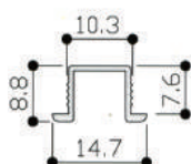
U型上軌 材質：鋁合金 顏色：鋁本色、古銅、金色
