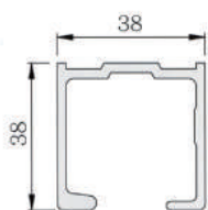
T.K. 藍白輪 軌道
