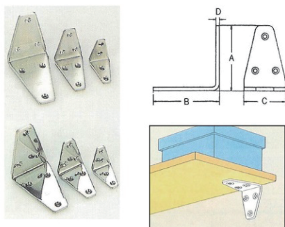
CH7322不銹鋼L型固定器
