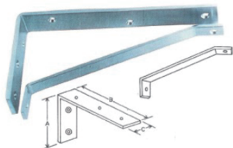
7325不銹鋼三角架(重型)
