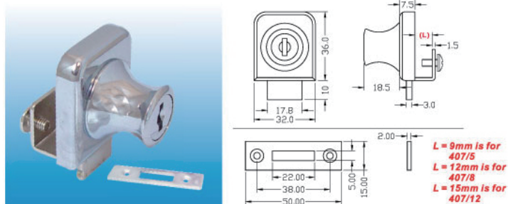
407 玻璃鎖(5、8、12)
