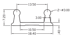
輪子(有邊蓋)
