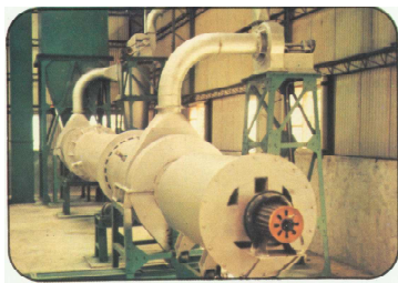
Double Tube Rotary Dryer 雙管迴轉式乾燥系統
